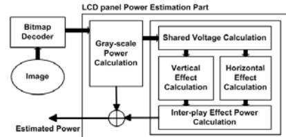
그림 3. LCD 패널 전력 소모 예측 시뮬레이터 구조
